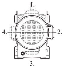
Klemens Pozisyonları Terminal Box Positions Klemenskasten Positionen
